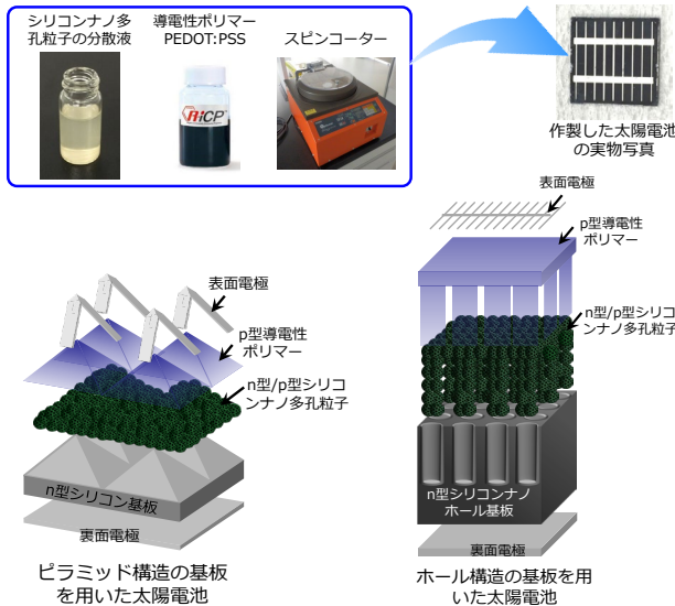
図5 太陽電池の構造図
