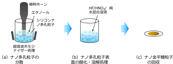
図3 n型/p型Siナノ金平糖粒子の製造プロセス
