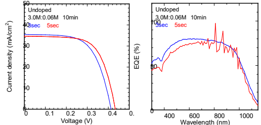
図6 各種太陽電池のJ-V特性と量子効率
